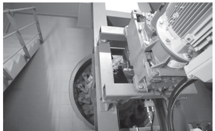
Eine Turbine leitet die kinetische Energie des fließenden Rems-Wassers an den Generator weiter, der sie in elektrische Energie umwandelt. (Bild: REMSTALWERK)
